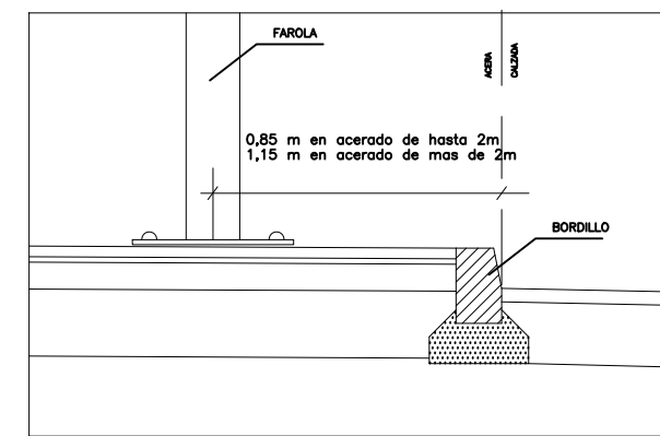
DETALLE COLOCACIÓN DE FAROLAS
