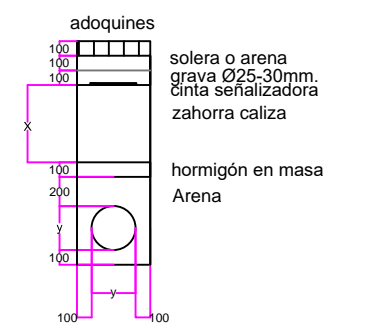
ZANJA TIPO
