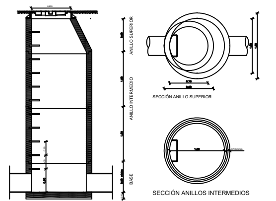
POZO DE REGISTRO CIRCULAR PREFABRICADO Ø1m
