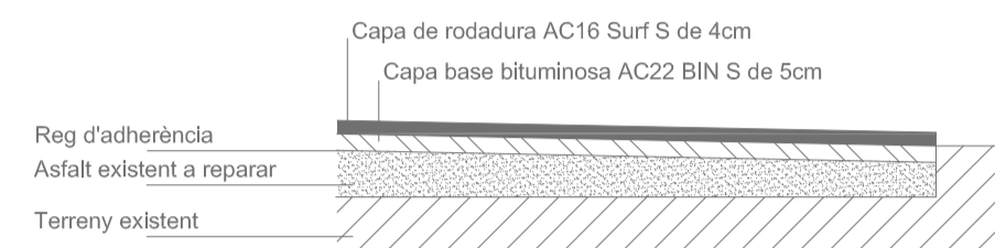
SECCIÓ A e:1/25
